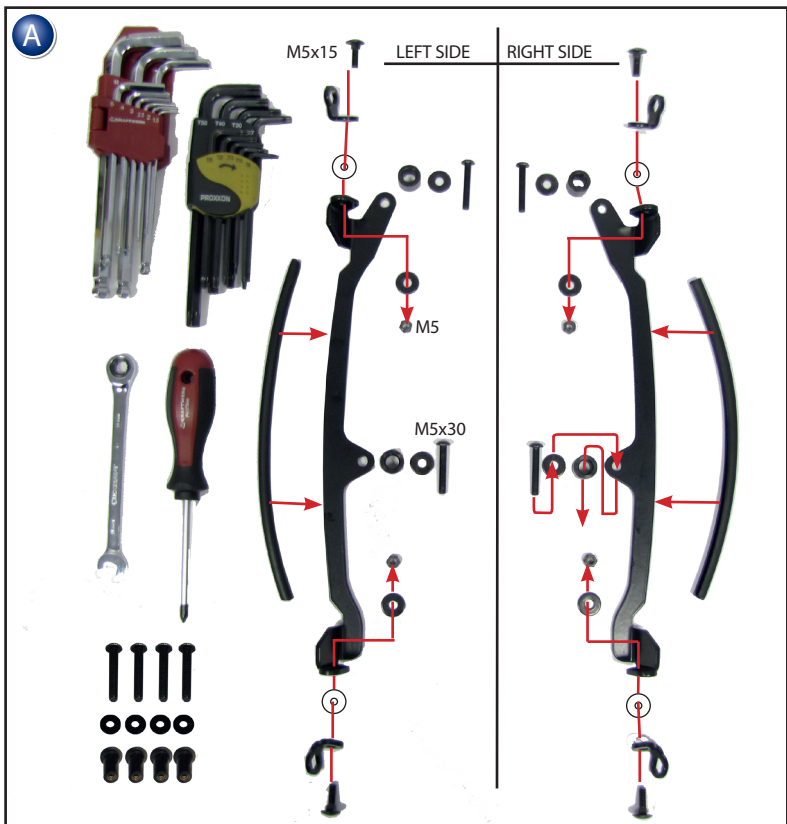
„CLEAR PROTECT“ Beinschützer BMW K 1600 GT/GTL Bestellnummer 35400
