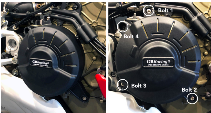
Bolt 3 M6X40A2-TORX - 10Nm
